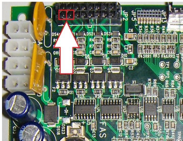
Détail connecteur JP2
